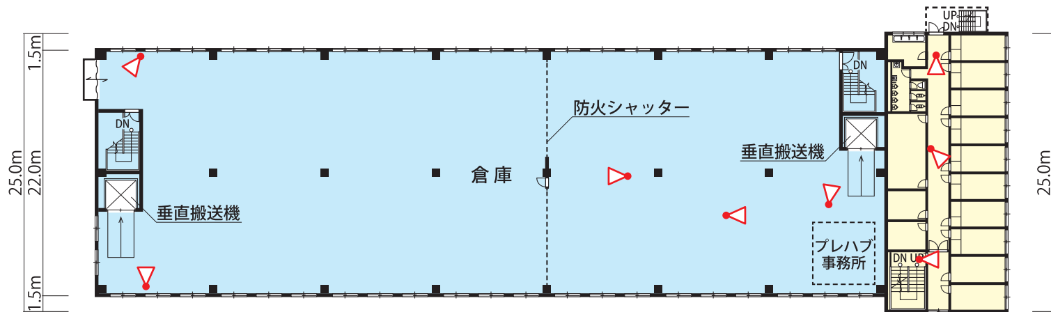
【2階平面図】
