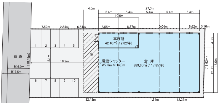
【配置平面図】
